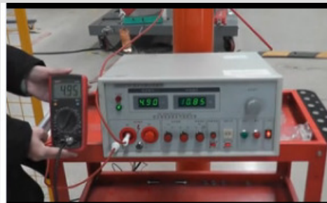
HV tester
